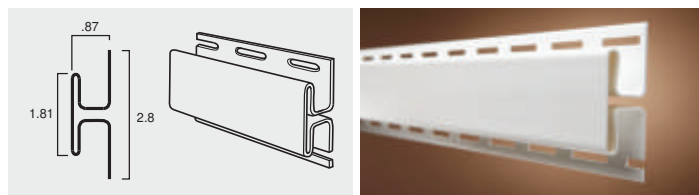
H-TRIM
