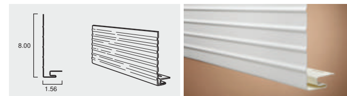
FASCIA-J
